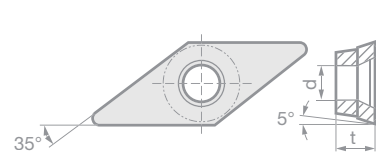
Rys. Płytki VBMT
