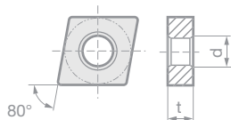
Rys. Płytki CNMG
