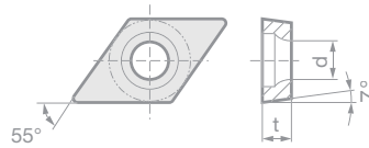
Rys. Płytki DCMT
