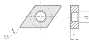
Rys. Płytki DNMG
